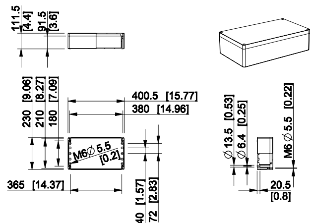
Ensto Cubo H 230 x 400,5 x 111,5 mm
